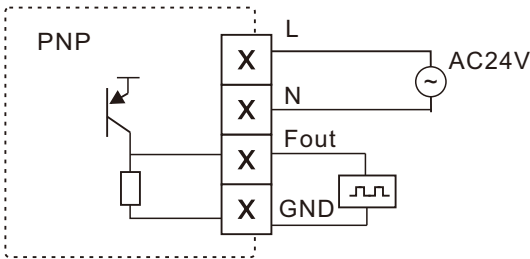
图5-10脉冲/脉冲当量输出接线图
