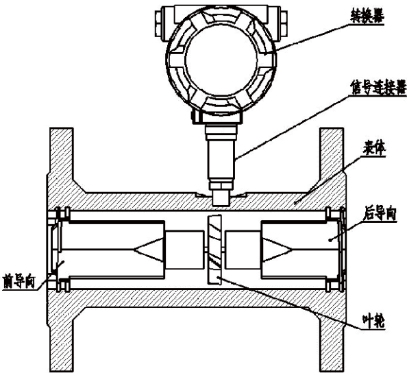
图1-1 法兰型涡轮流量计结构图
