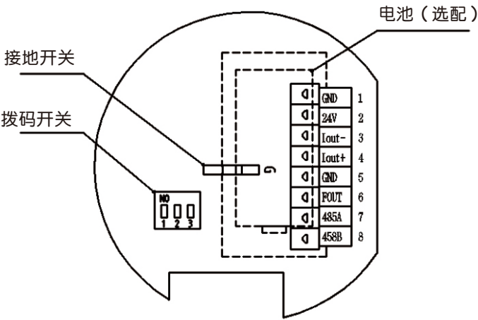
图5-3 DC24V供电端子板
