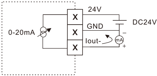
图5-7 三线0-20mA输出接线图
