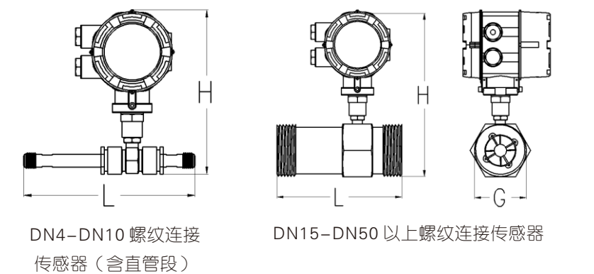
图4-1 螺纹连接示意图
