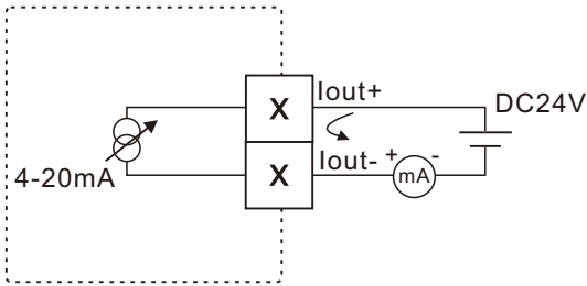
图5-5 两线制4-20mA输出接线图
