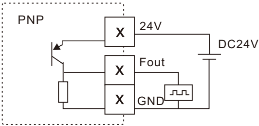
图5-4 脉冲/当量脉冲输出接线图
