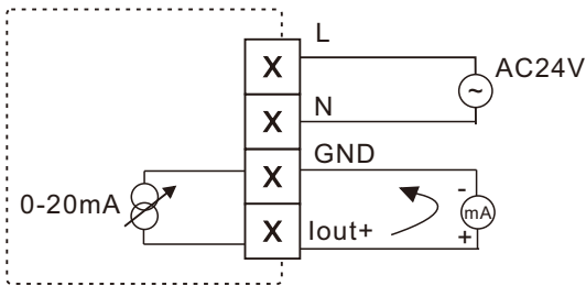
图5-12 四线制0-20mA接线图
