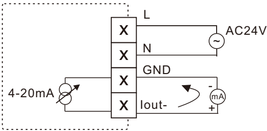
图5-11 四线制4-20mA接线图
