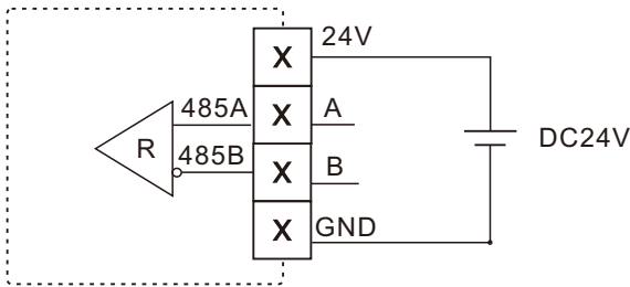
图5-8 RS485输出接线图
