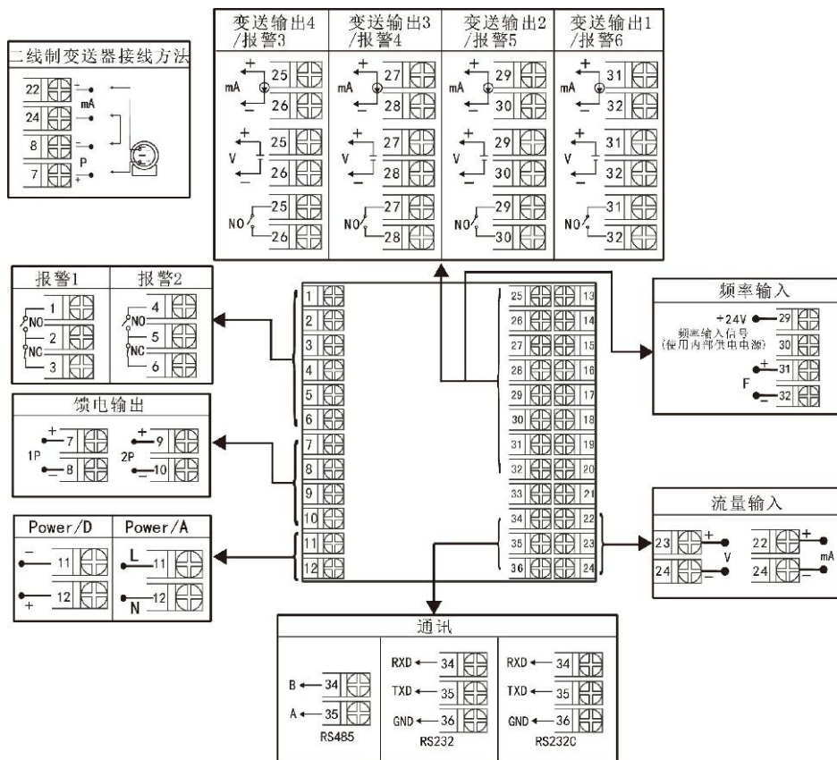
NHR-7601/7601R 系列接线图
